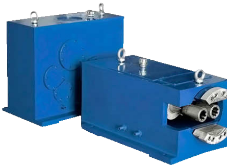
REDUTOR ROSCA SEM-FIM
